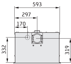
Maattekening van boven
