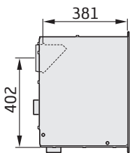
Rookuitgang naar achteren Aansluitstuk Ø125 mm
