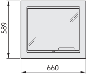
Omlijsting en deur van glas
